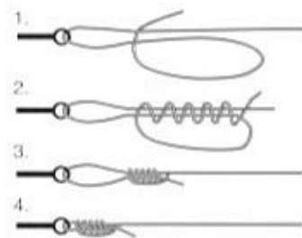
Kuva 4: Koukkusolmu
